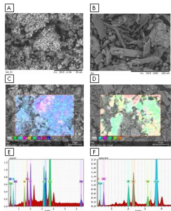
Figura 1. Análises morfológicas: (A) MEV farinha de osso in natura; (B) MEV hidroxiapatita in natura; (C) MEV farinha de osso após 30 min em contato com a solução; (D) MEV hidroxiapatita após 30 min em contato com a solução; (E) EDS da farinha de osso após o processo de biossorção; (F) EDS da hidroxiapatita após o processo de biossorção.
